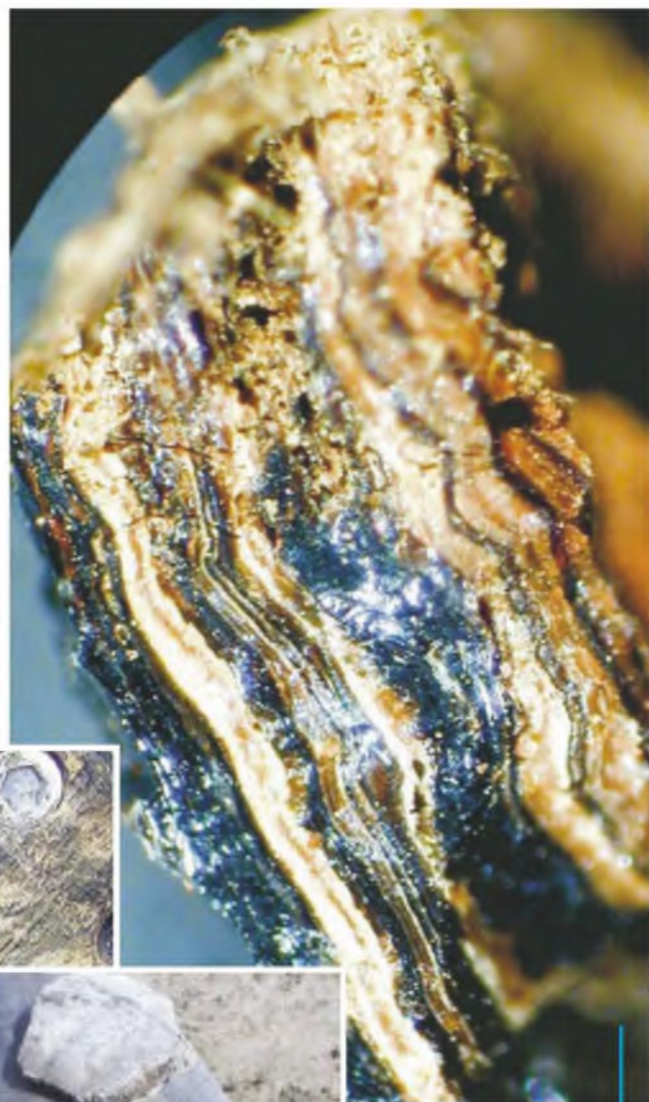
Вид слоев кристаллов под микроскопом (струвит) [\text{Mg}(\text{NH}_4)(\text{PO}_4) \cdot 6\text{H}_2\text{O}] .
